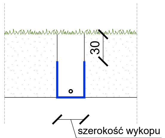
UKŁADANIE MATY NA TERENACH ZIELONYCH
