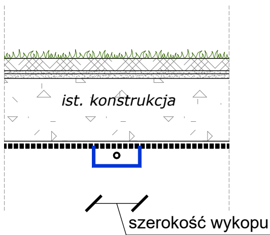
UKŁADANIE MATY POD KONSTRUKCJĄ PARKINGU/DROGI
