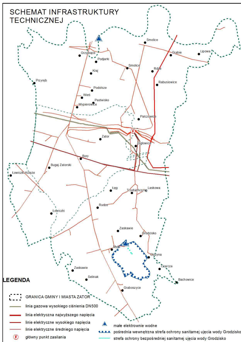
Ryc.35. Schemat infrastruktury technicznej na obszarze gminy Zator
