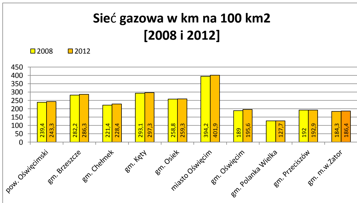
Ryc.41. Długość sieci gazowej na 100 km 2 Źródło: Opracowanie własne na podstawie danych GUS, 2012
