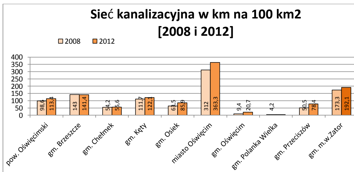
Ryc.39. Długość sieci kanalizacyjnej na 100 km 2 Źródło: Opracowanie własne na podstawie danych GUS, 2012
